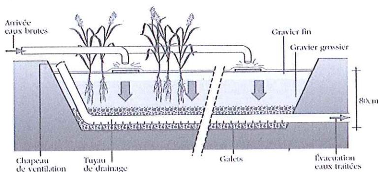
FILTRE VERTICAL : ALIMENTATION INTERMITTENTE AVEC AÉRATION PAR LA SURFACE
